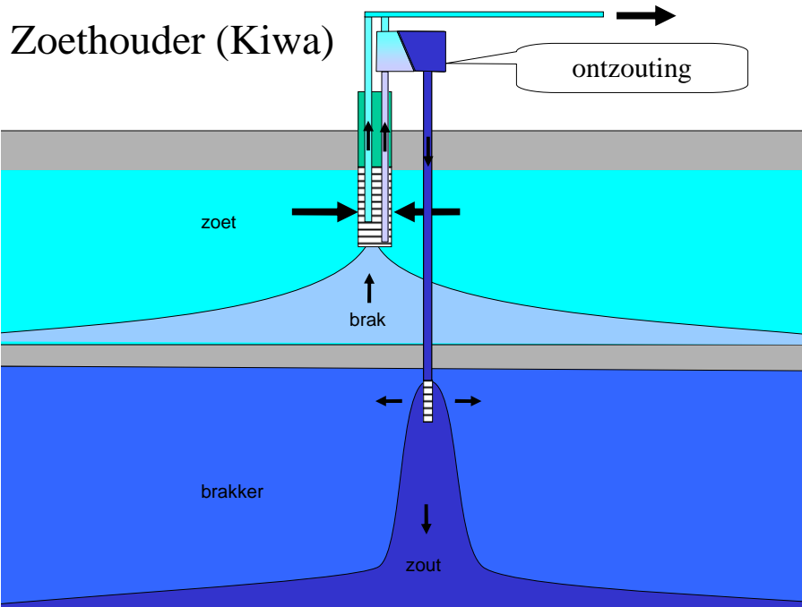
Figuur 7: Schematische voorstelling van de “zoethouder” waarbij echter gebruik wordt gemaakt van de hoge dichtheid om het het concentraat naar de basis van het watervoerend pakket te laten zinken.
