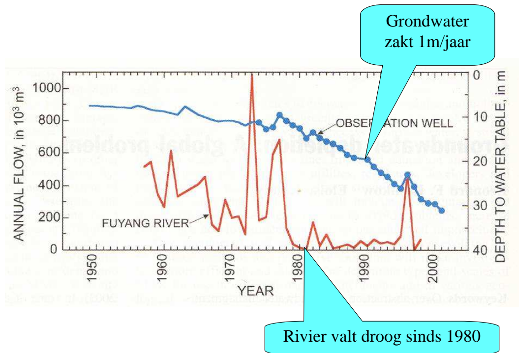
Figuur 3: Snelle grondwater daling in een put in Noord China, correlatie met droogvallen van de Fuyang Rivier (uit Konikow en Kandy, 2005, Hydrogeology Journal, 13: p319. Theme Issue on the Future of Hydrogeology.
