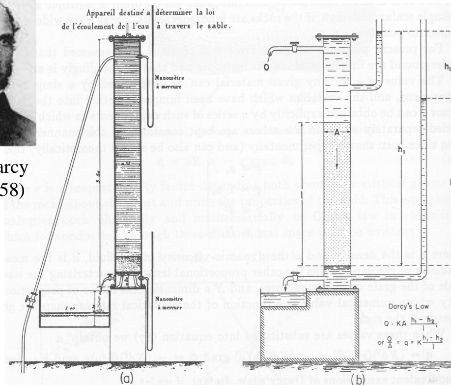
Figuur 1: Henry Darcy met zijn oorspronkelijk meetopstelling en de meer schematische tekening uit Hubbert (1940)
