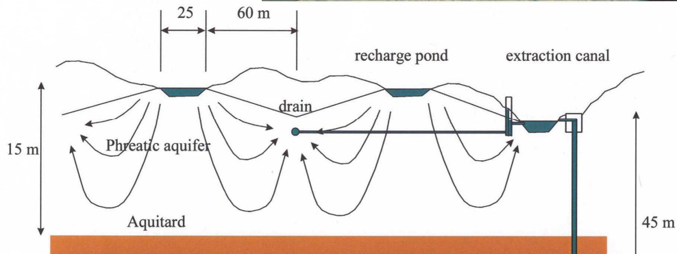
Figuur 4: Kunstmatige infiltratie in de Amsterdamse Waterleidingduinen ten zuiden van Zandvoort. Het geïnfiltreerde voorgezuiverde rivierwater stroomt in gemiddeld 3 maanden naar de “drains” en de onttrekkingskanalen.
