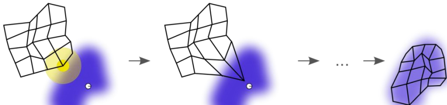
Afbeelding 4 Illustratie van het trainen van een Self-Organizing Map. De blauwe polygoon representeert de invoergegevens, het witte raster de neuronen die zich initieel willekeurig in de ruimte bevinden. Na een aantal iteraties zal het raster van neuronen de structuur van de data vertegenwoordigen.
