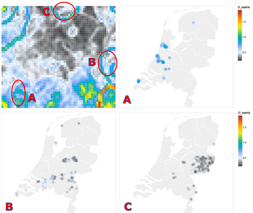
Afbeelding 12 U-matrix als resultaat van SOM. Er zijn drie voorbeelden van clusters geselecteerd waarvan de locaties van de onderliggende data gevisualiseerd zijn in a), b) en c), respectievelijk.
