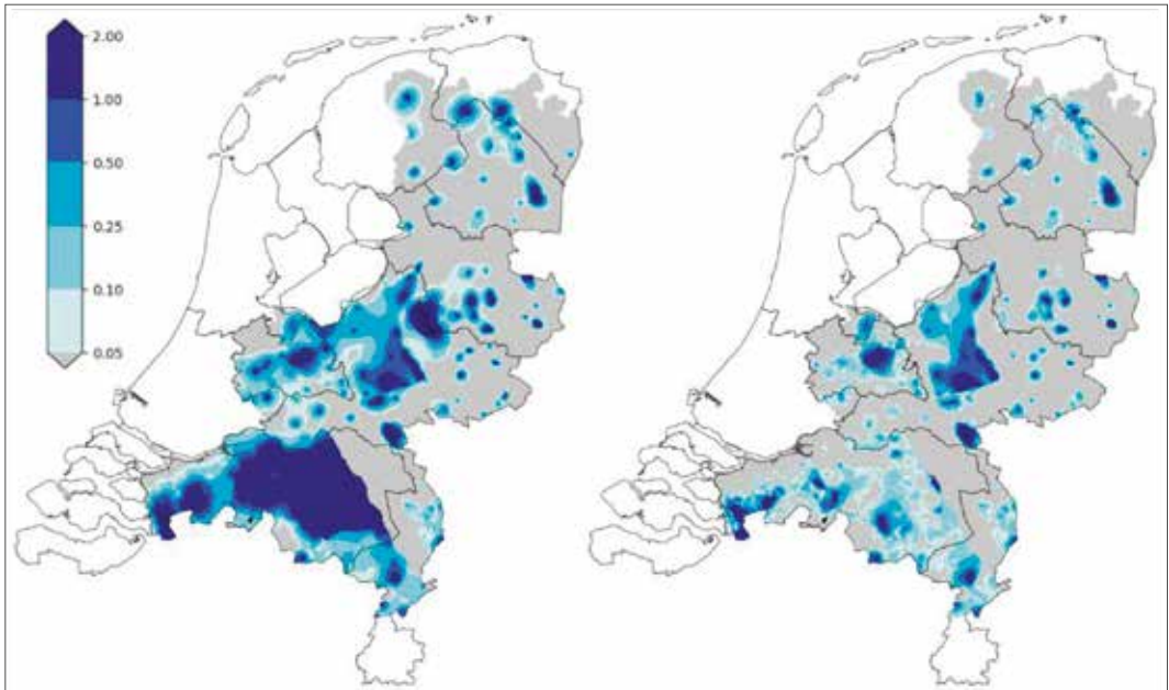
Afbeelding 3 Het berekende effect op de stijghoogte (links) en de freatische grondwaterstand (rechts) voor de zomersituatie (LG3) in 2018, 5,5 jaar na volledig stopzetten van de drinkwaterwinning op 1 januari 2013.
